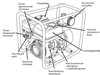
Внешний вид спереди
